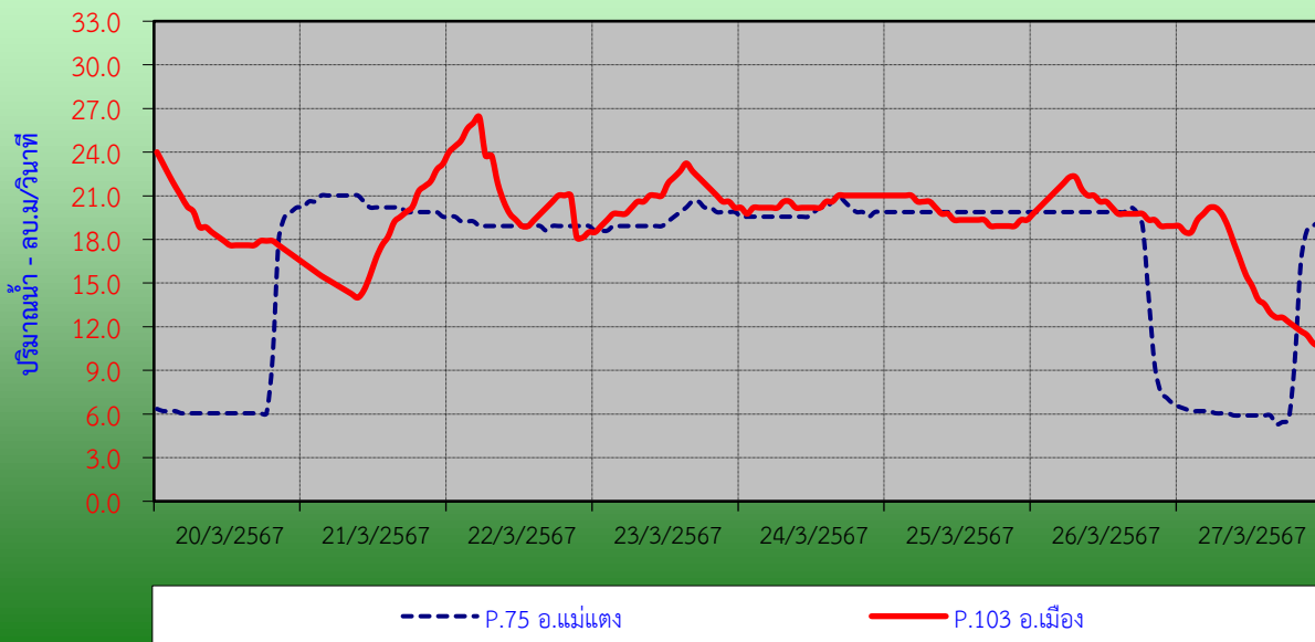
กราฟแสดงปริมาณน้ำปิ้งรายชั่วโมงรอบวันที่ 12/2567 ที่สถานีแม่ น้ำปิ้ง ( P.75) บ้านซ้อแล อ.แม่แตง และที่สถานีแม่ น้ำปิ้ง (P.103) บ้านป่าซ่อยใต้ อ.เมือง จ.เชียงใหม่
